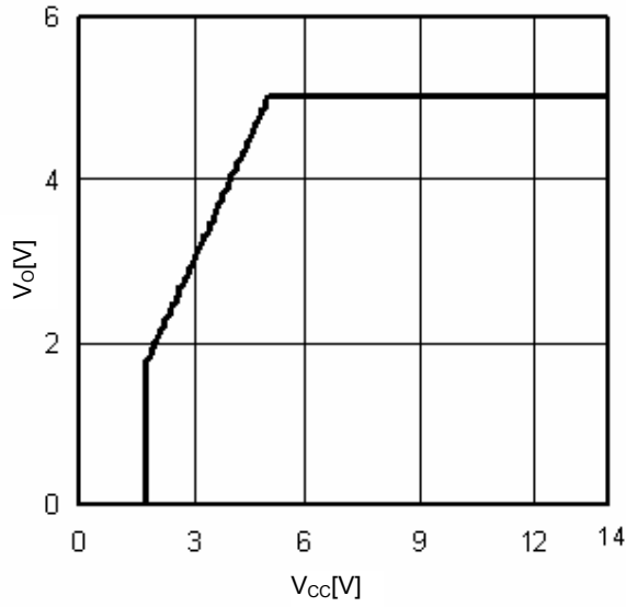
Fig.15 V_{cc}-V_o ( I_o=0mA )
