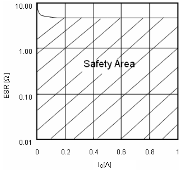
Fig.19 ESR condenser
