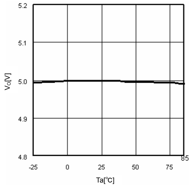
Fig.9 T_a-V_O ( I_o=0mA )
