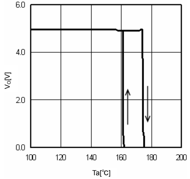
Fig.16 TSD ( I_o=0mA )
