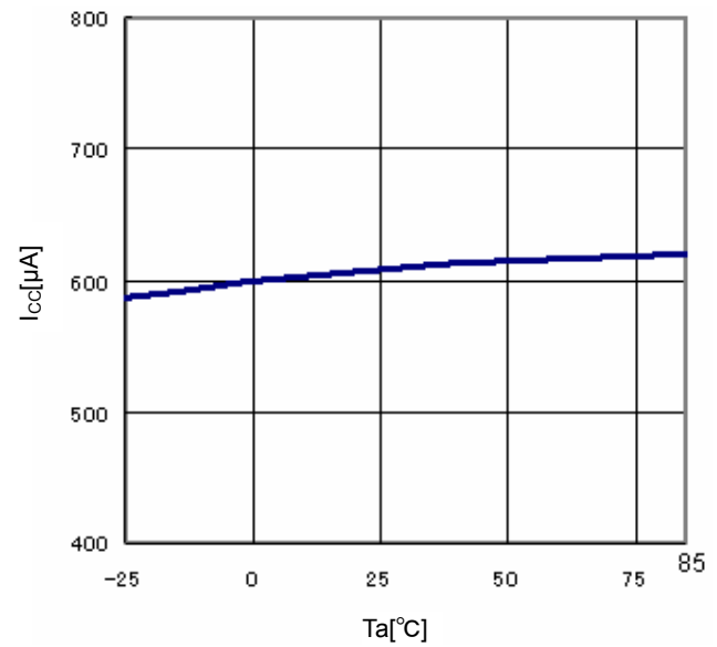
Fig.10 T_a-I_{cc}
