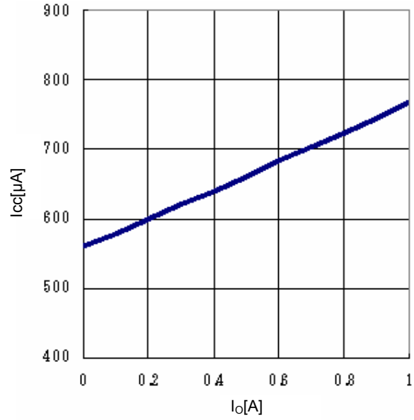
Fig.20 I_o - I_{cc}
