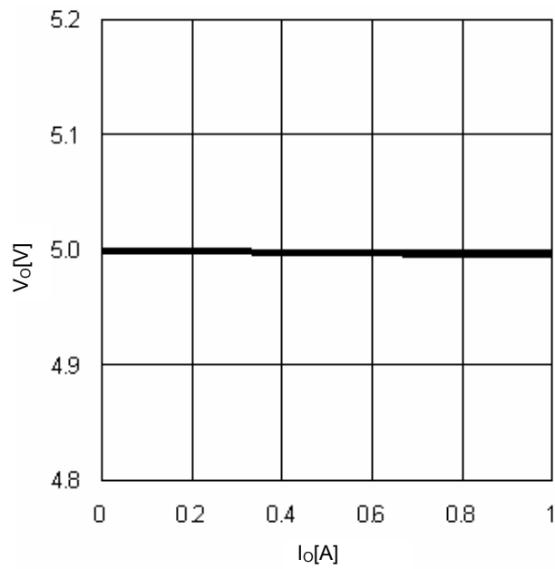
Fig.13 I O -V O
