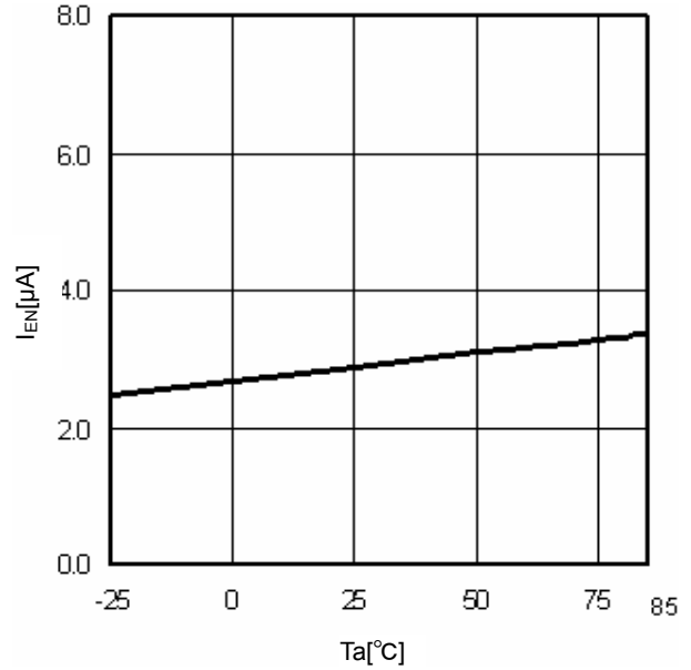
Fig.12 T a -I EN
