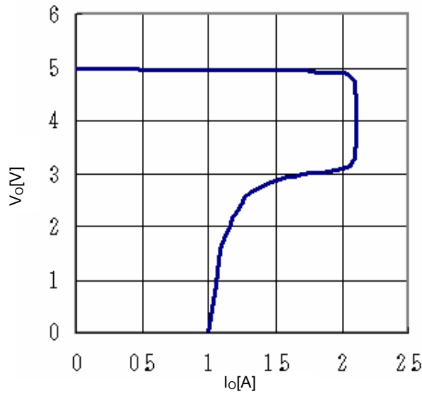
Fig.17 OCP
