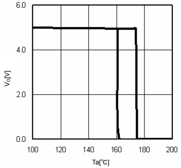
Fig.16 TSD (I o =0mA)
