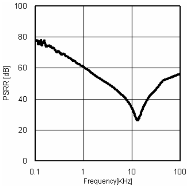
Fig.21 PSRR(Io=0mA)
