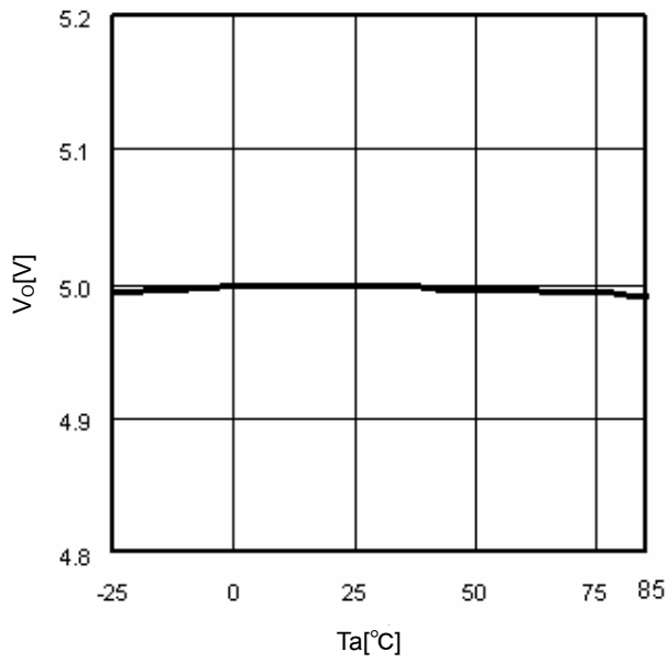
Fig.9 T_a-V_O ( I_o=0mA )
