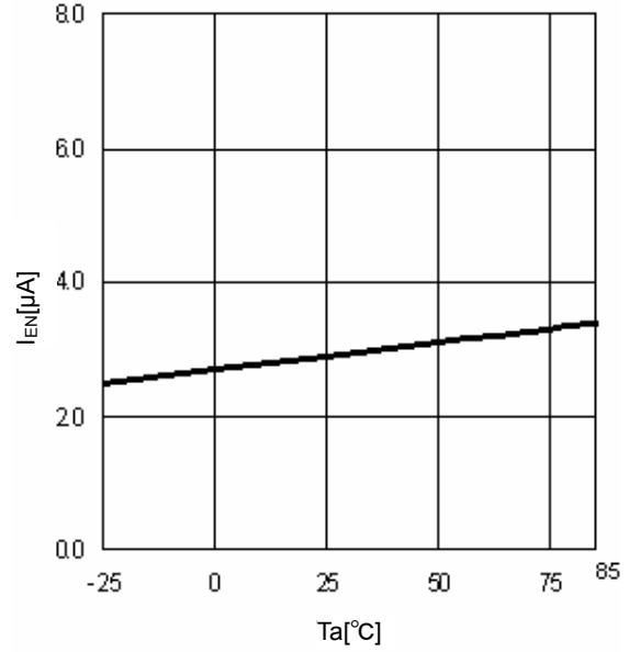
Fig.12 T_a - I_{EN}
