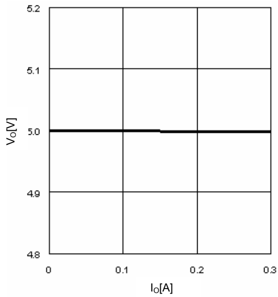
Fig.13 I_O - V_O
