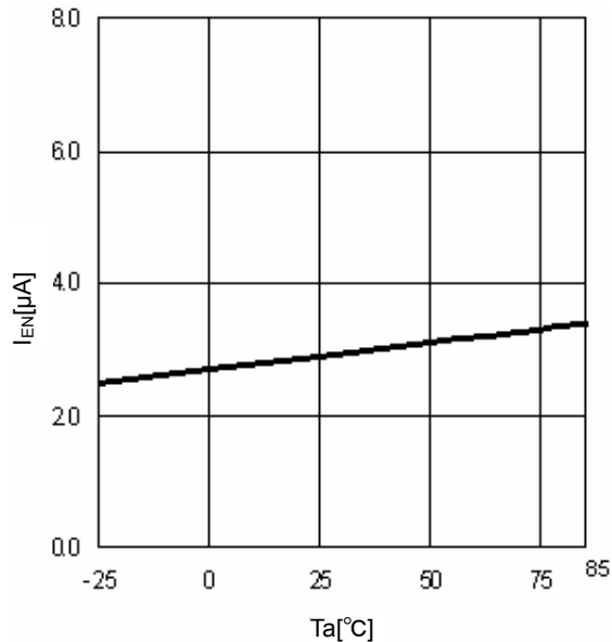
Fig.12 T_a - I_{EN}
