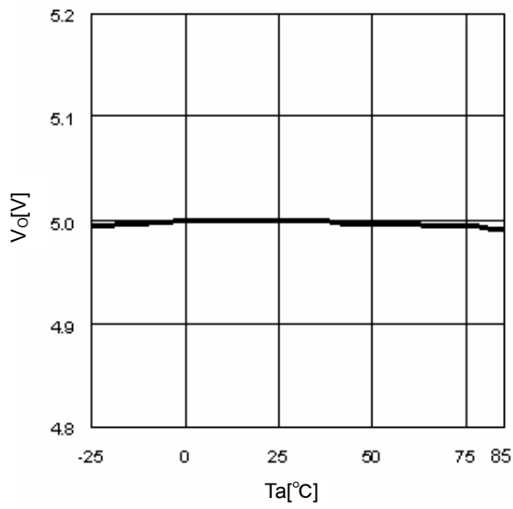
Fig.9 Ta-V O (I O =0mA)
