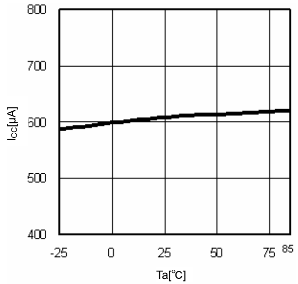
Fig.10 Ta-I cc
