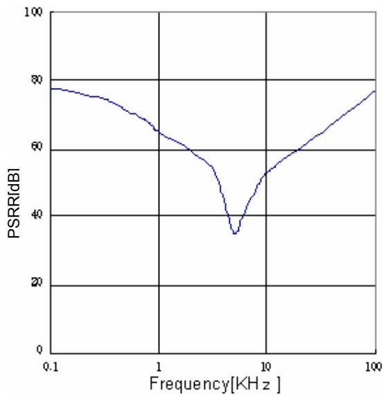
Fig.21 PSRR( I_o=0mA )
