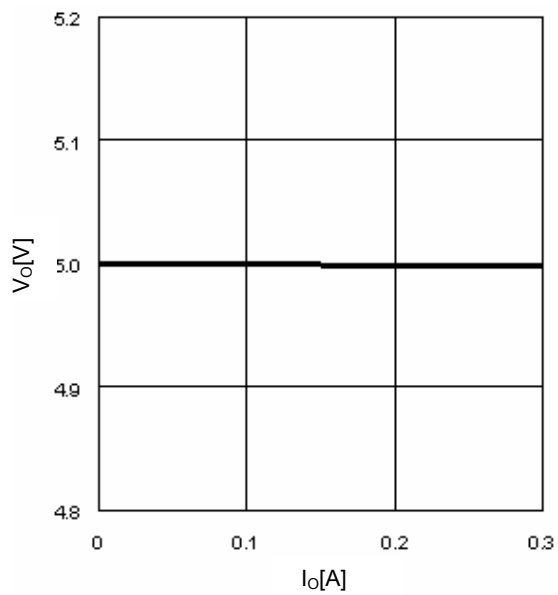
Fig.13 I_O - V_O
