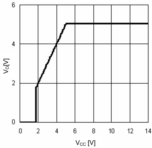
Fig.15 V_{CC}-V_O ( I_o=0mA )
