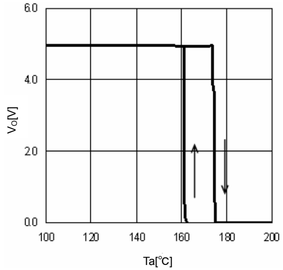
Fig.16 TSD ( I_o=0mA )
