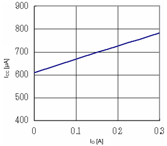
Fig.20 I_o - I_{cc}
