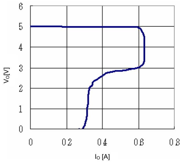
Fig.17 OCP
