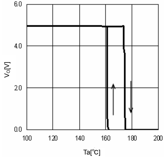
Fig.16 TSD (I O =0mA)
