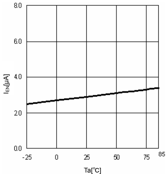
Fig.12 T_a - I_{EN}
