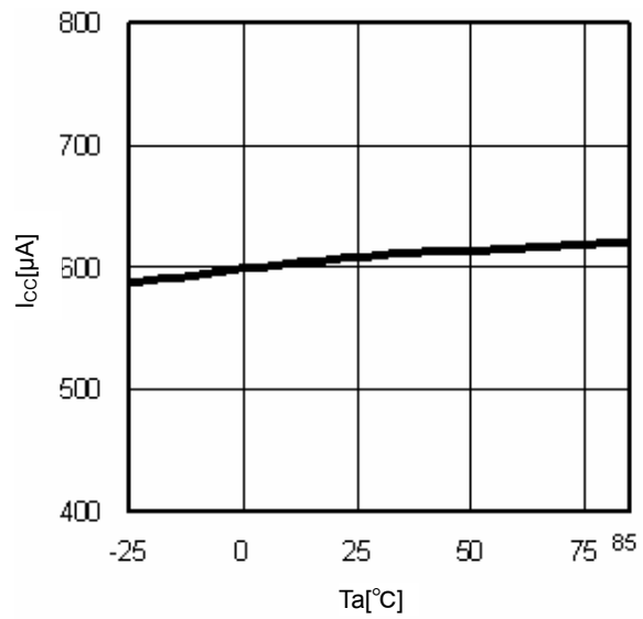
Fig.10 Ta-I cc
