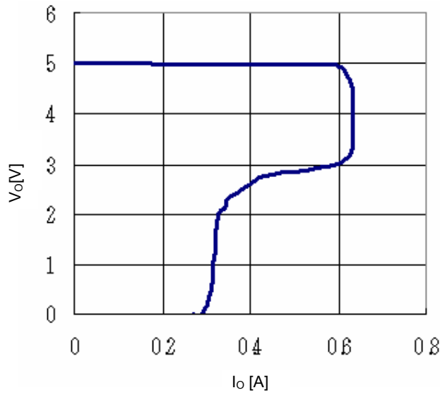
Fig.17 OCP
