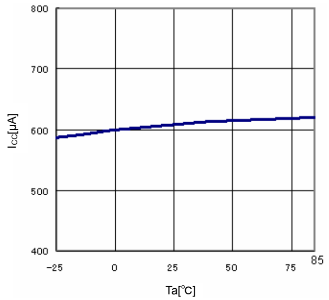
Fig.10 T_a-I_{cc}
