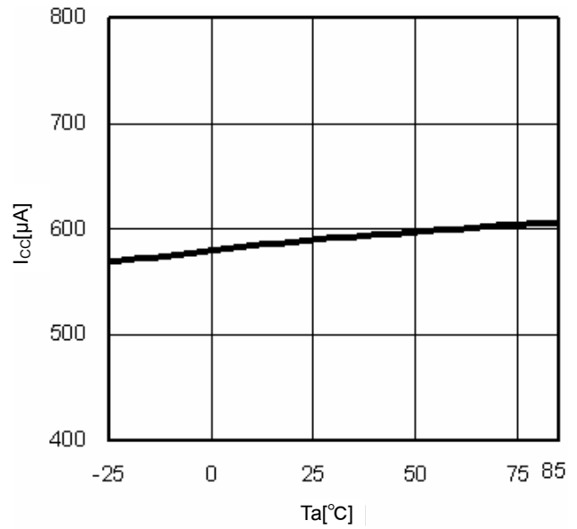
Fig.10 Ta-I cc
