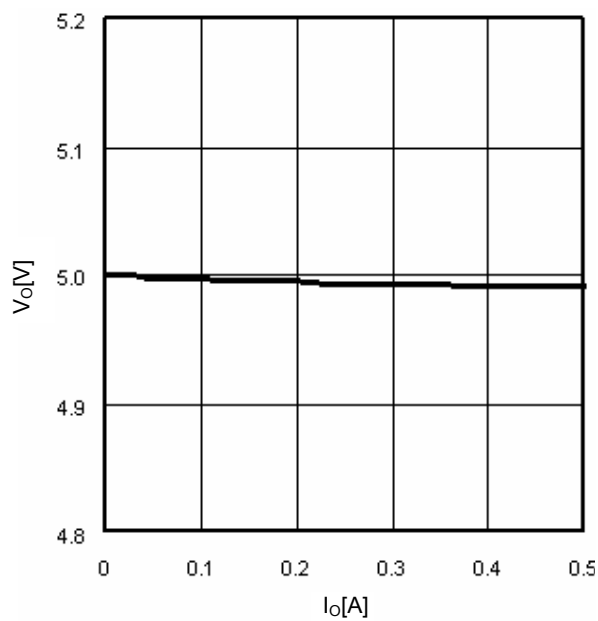
Fig.13 I_o - V_o
