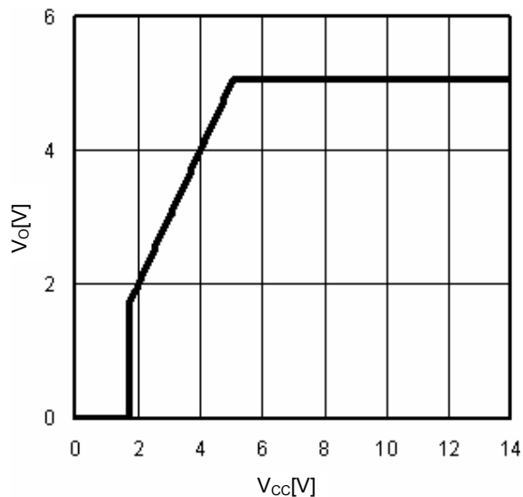
Fig.15 V_{cc}-V_o ( I_o=0mA )
