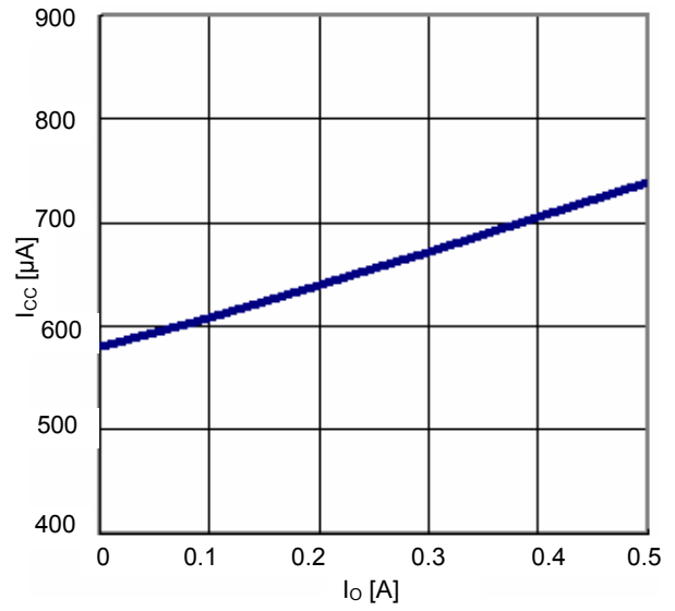
Fig.20 I_o - I_{cc}
