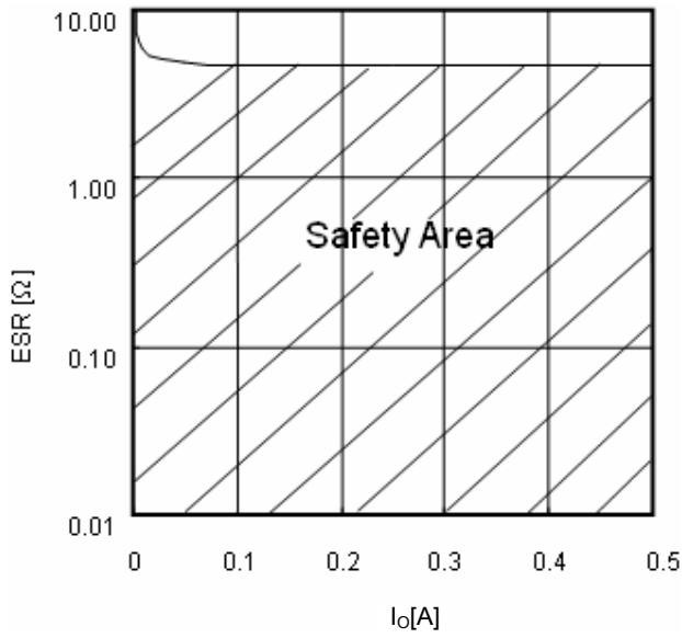
Fig.19 ESR condenser
