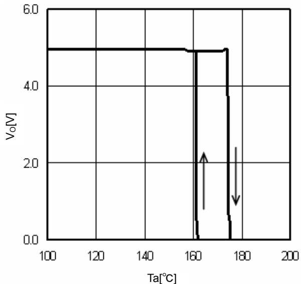
Fig.16 TSD ( I_o=0mA )
