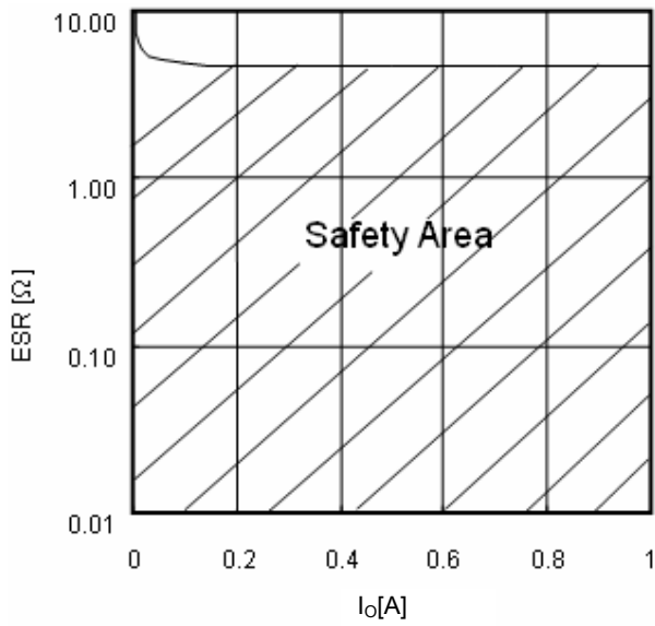
Fig.19 ESR condenser
