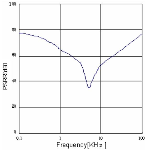
Fig.21 PSRR( I_o=0\text{mA} )
