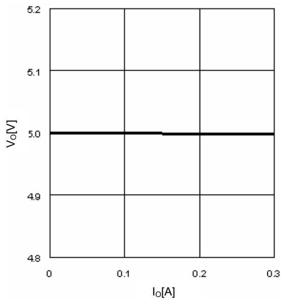
Fig.13 I_O - V_O
