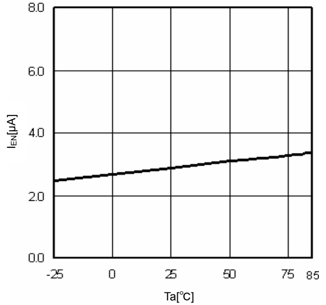
Fig.12 T_a - I_{EN}
