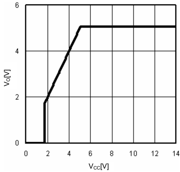
Fig.15 V_{cc}-V_o ( I_o=0mA )
