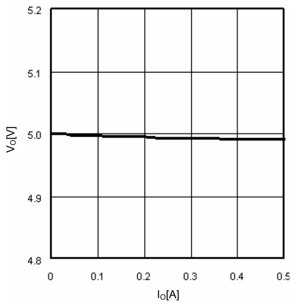
Fig.13 I_o - V_o
