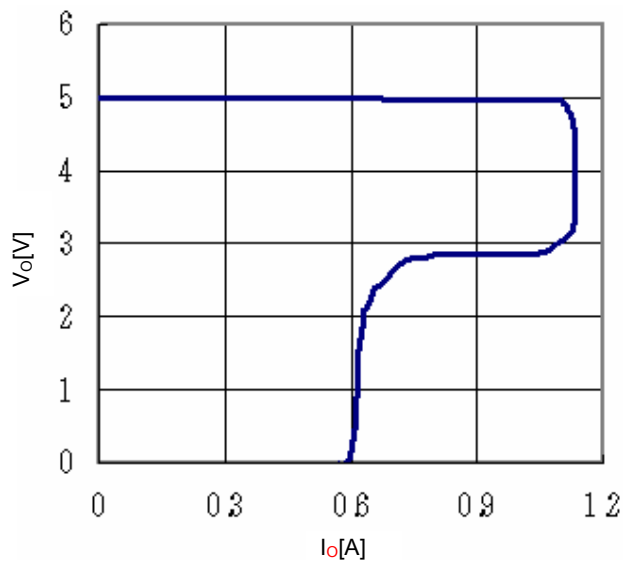
Fig.17 OCP
