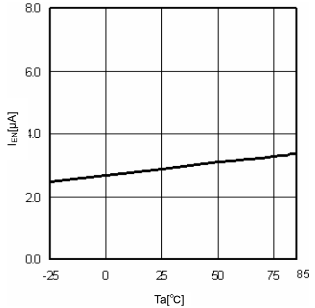
Fig.12 T_a - I_{EN}
