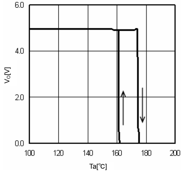
Fig.16 TSD ( I_o=0mA )
