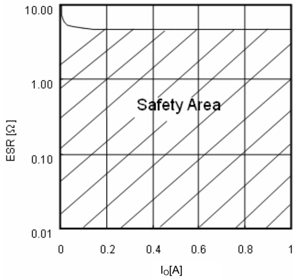
Fig.19 ESR condenser
