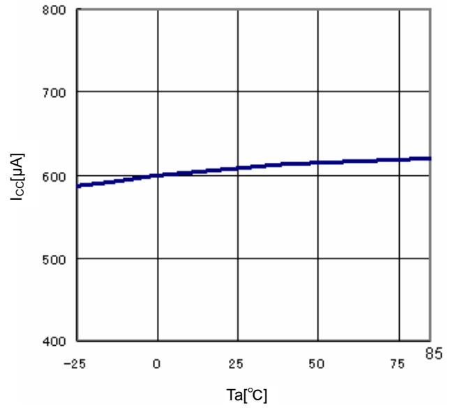
Fig.10 T_a-I_{cc}
