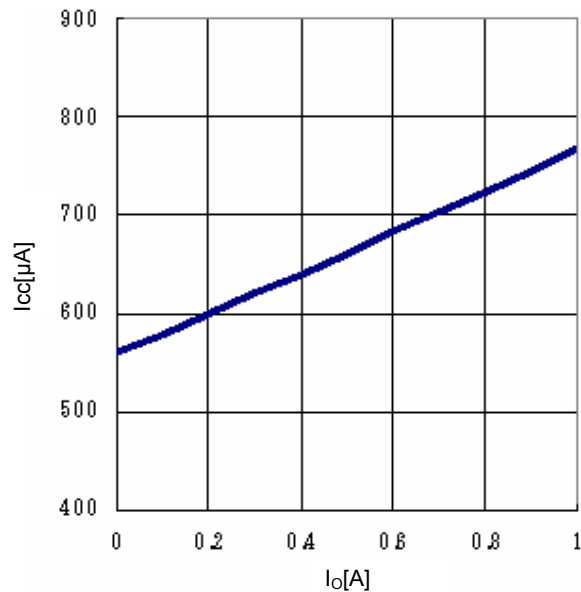
Fig.20 I_o - I_{cc}
