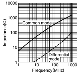
ACM2520-102-2P
