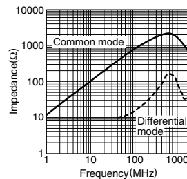
ACM2520-801-3P
