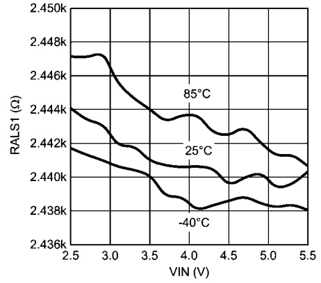
ALS Resistance vs VIN R_{ALS1} , (2.44k \Omega setting)
