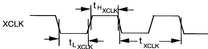
Fig. 25 XCLK=37.056MHz Input Timing
