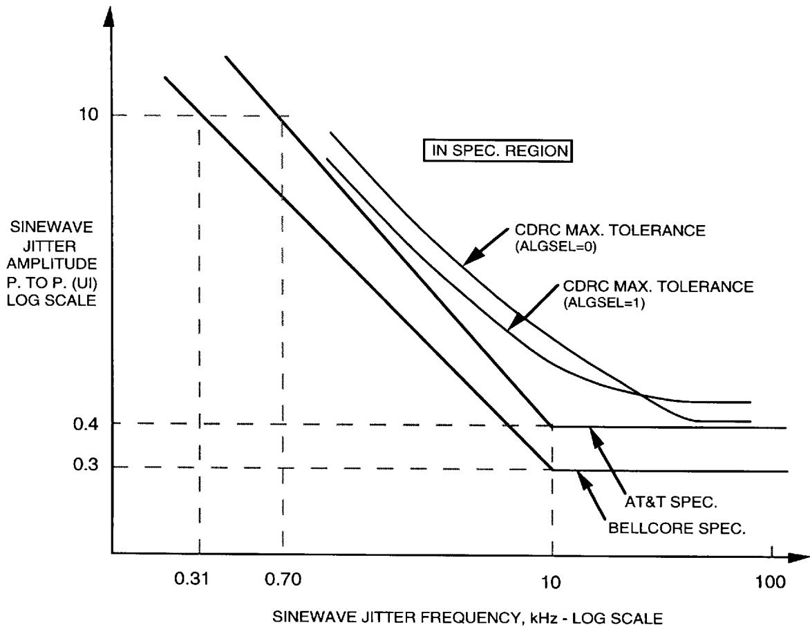
Fig. 2 CDRC Jitter Tolerance
