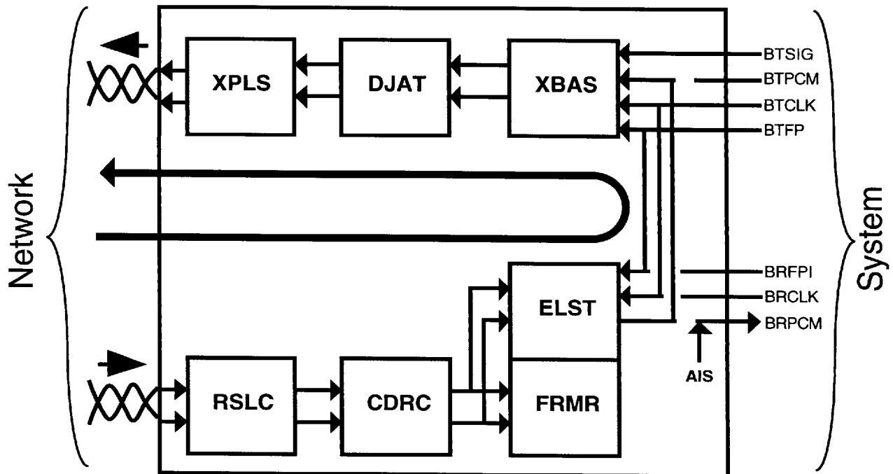
Fig. 8 Payload Loopback
