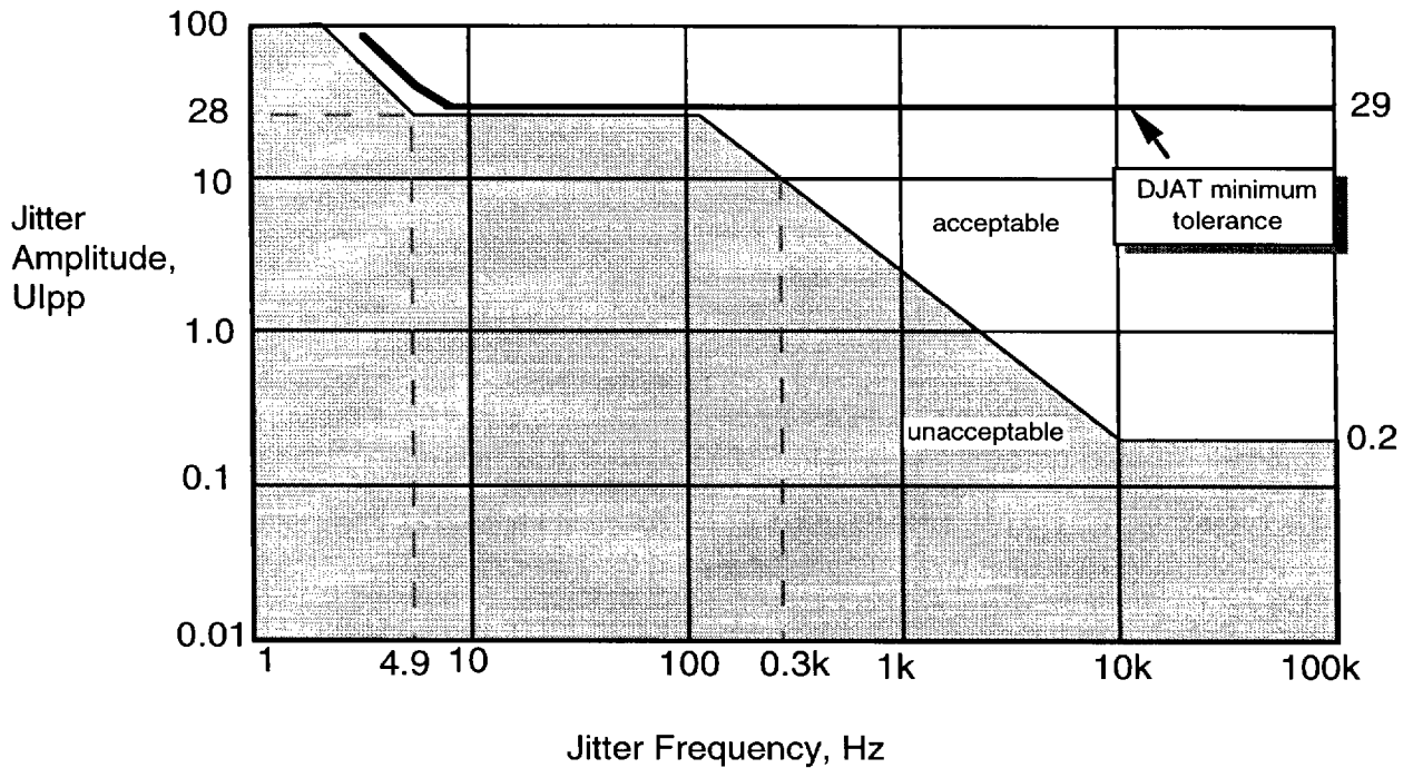
Fig. 3 DJAT Jitter Tolerance
