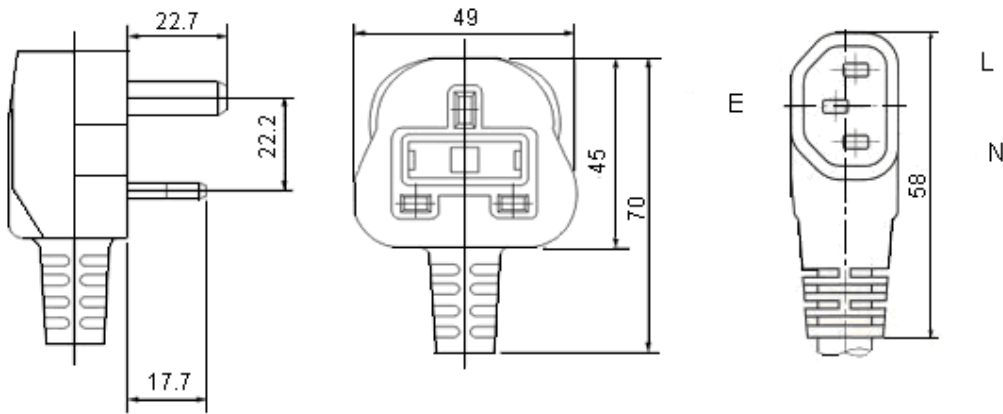
Dimensions : Millimetres
