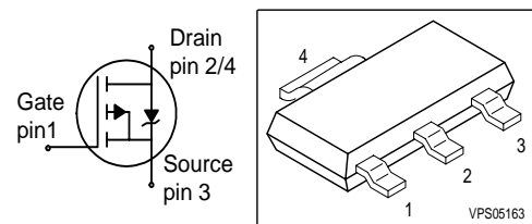
PG-SOT-223
