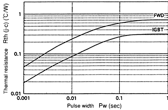
過渡熱抵抗特性 Transient thermal resistance
