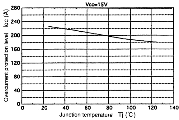
過電流保護—接合部温度特性
