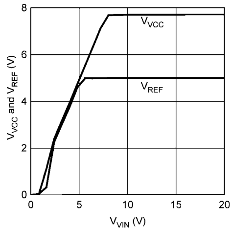
V VCC and V REF vs V VIN
