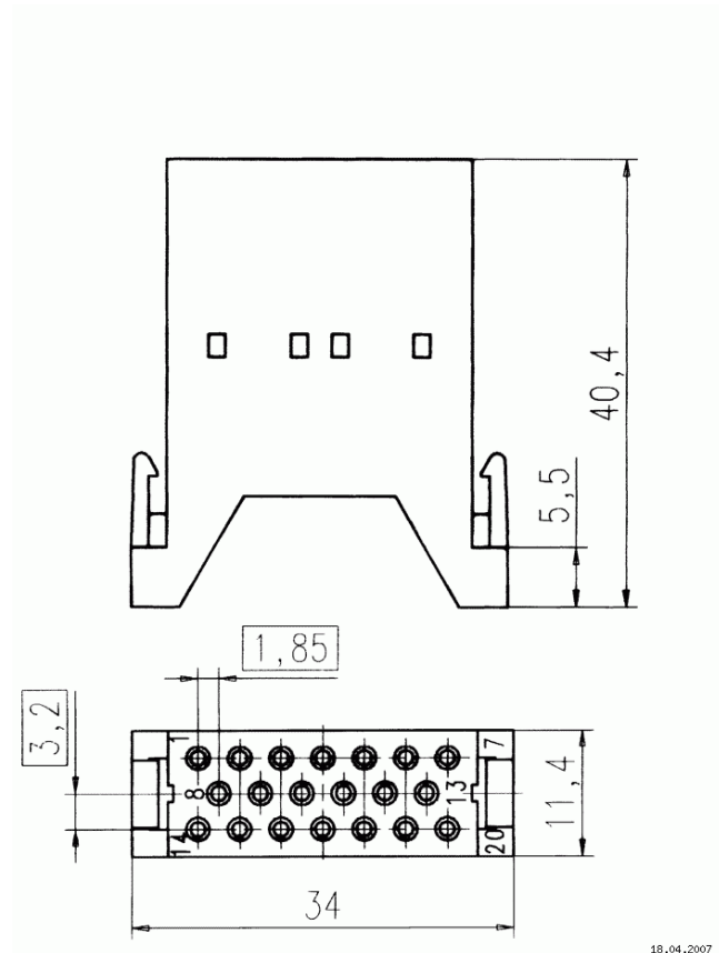
Maßzeichnung Dimensions in mm (Inch)
