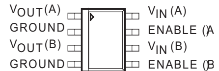
MIC5202-xxBM
