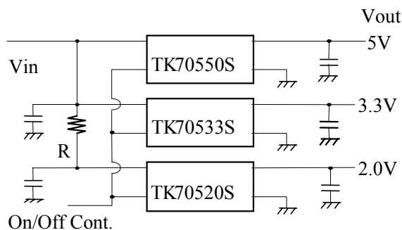
図13-4 並列接続例
