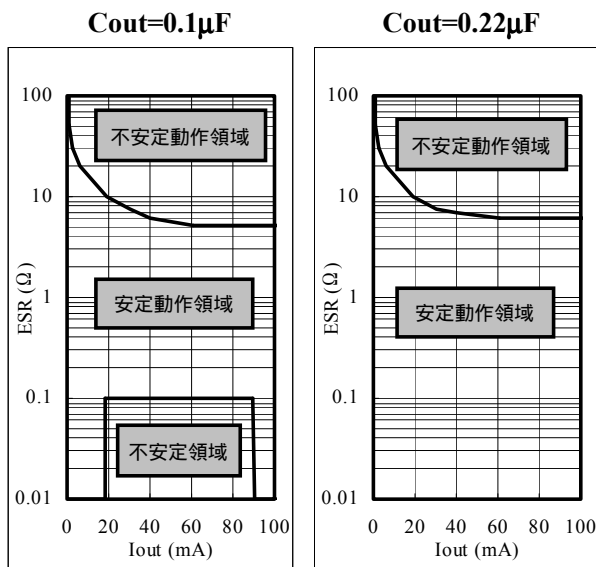
図13-2 安定動作領域特性
