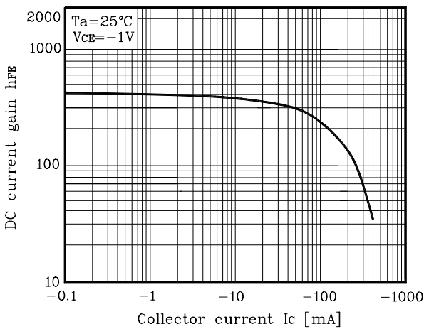
Fig. 3 h_{FE} - I_C
