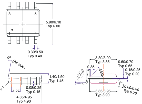
(4) SOP-8L
