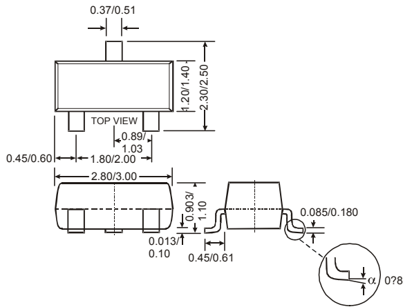
(3) SOT23
