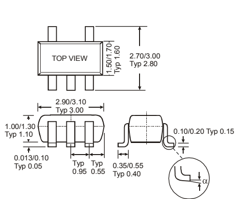
(1) SOT25
