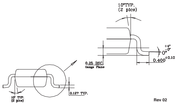
TSOT-23-5 (D5)
