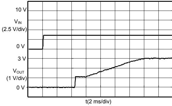
S-8520/1C30MC ( V_{IN} : 0 → 3.6 V)
