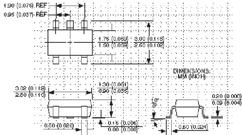
SOT-23-5 (M5)
