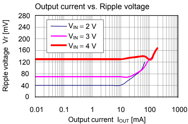
(5) S-8354A50MC
