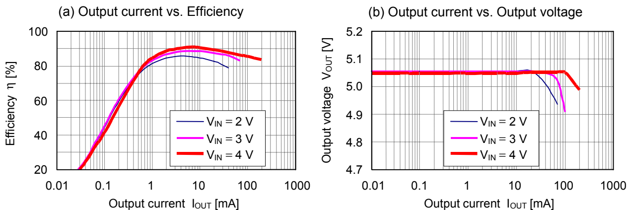
(3) S-8353H50MC
