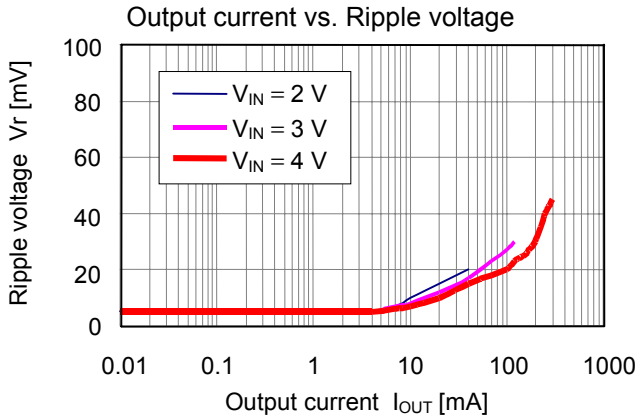
(3) S-8353H50MC
