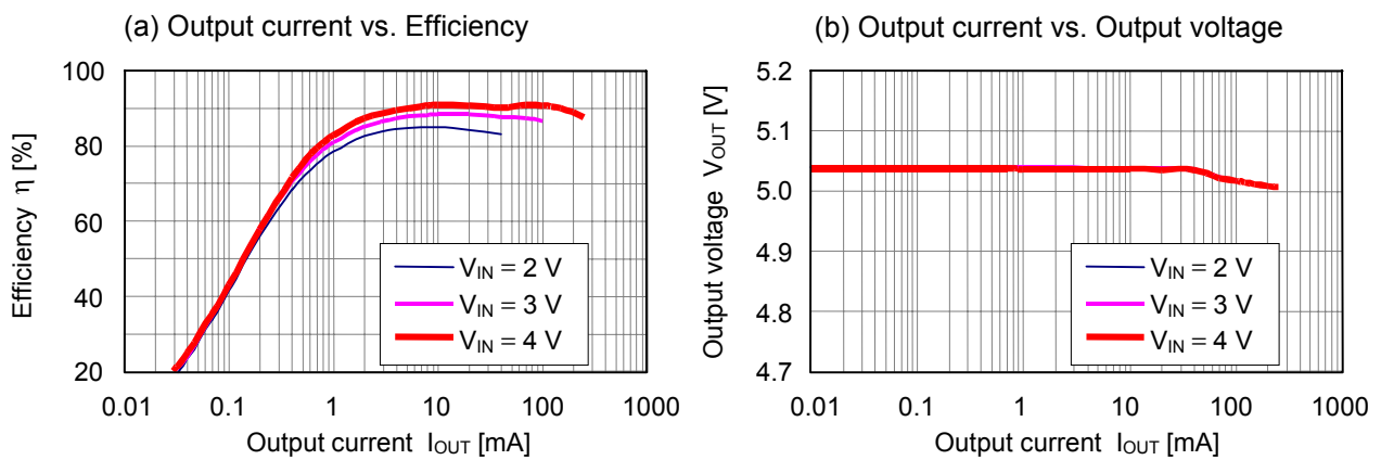
(2) S-8353H50MC
