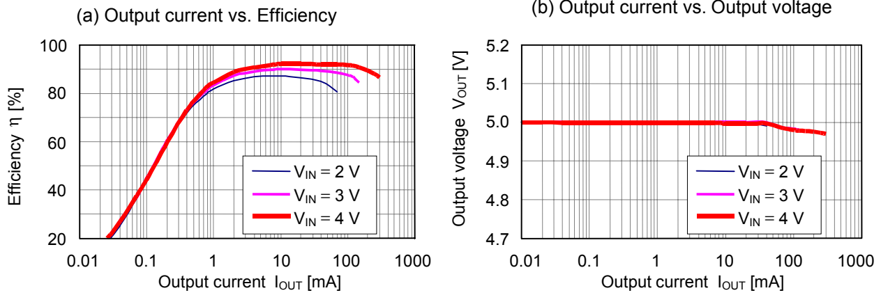
(2) S-8353H50MC
