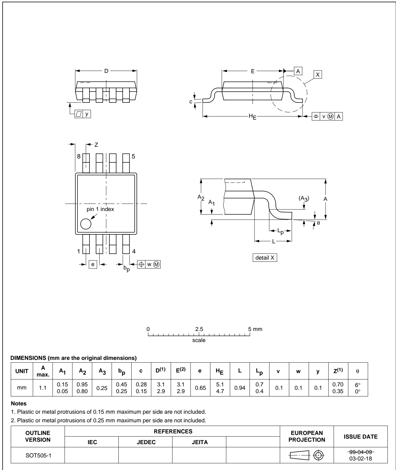
Fig 24. Package outline SOT505-1.
