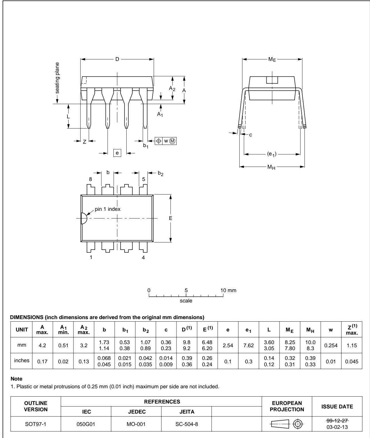
Fig 22. Package outline SOT97-1.
