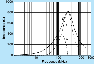
BLM21BD421SN1
