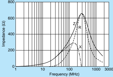
BLM21BD331SN1
