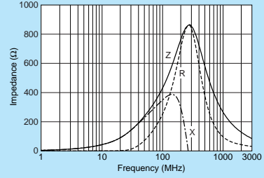
BLM18BD421SN1
