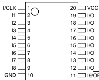
TSSOP
