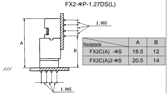
Receptacle
