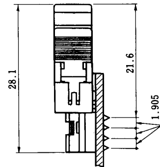
FX2B-*PA-1.27DS(L)
