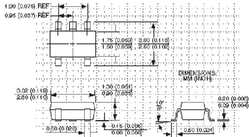
SOT-23-5 (M5)
