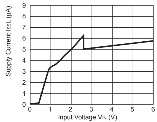
R1161x26xx (ECO=L)
