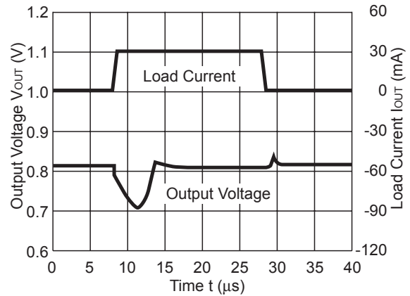
R1161x08xx (ECO=L)
