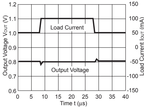
R1161x08xx (ECO=H)
