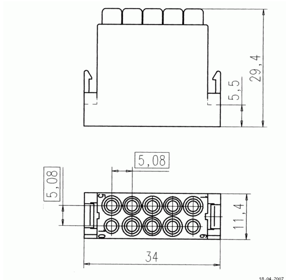
Maßzeichnung Dimensions in mm (Inch)
