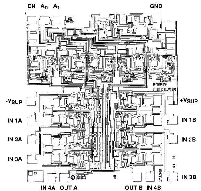
HI-509
