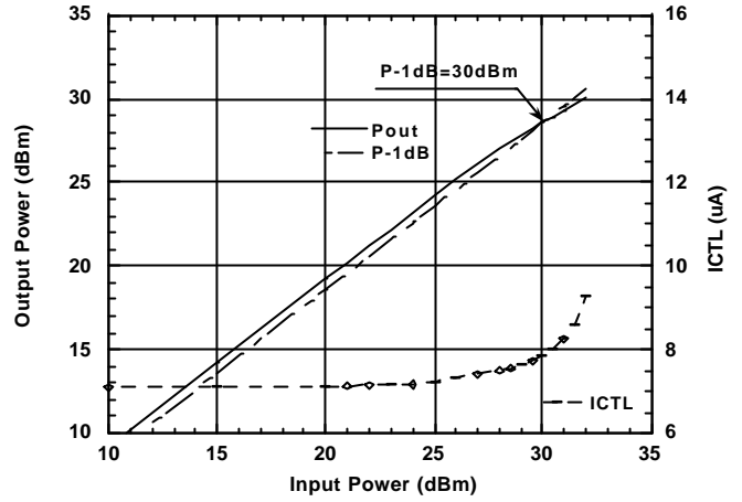
Input Power vs. Output Power, I_{CTL} (V_{CTL(L)}=0V, V_{CTL(H)}=2.7V)
