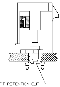
PRESS FIT RETENTION CLIP
