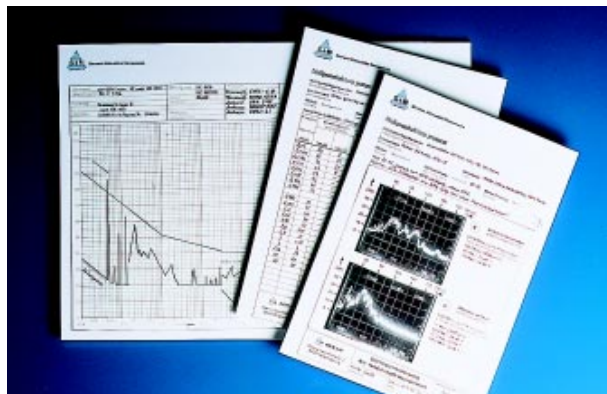
Störfeldstärkemessung mit Spectrum Analyzer und Meßempfänger Measuring radiated emission with spectrum analyzer and test receiver
