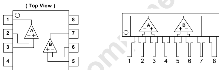
NJM4565L
