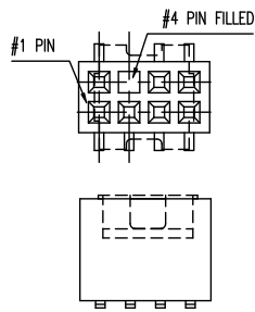
P/N: 20021321-00108D4LF
