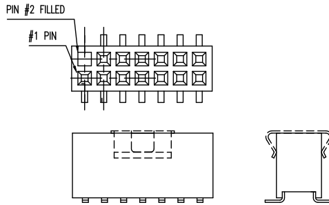
P/N: 20021321-00214D4LF
