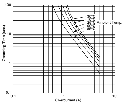
PTGL12AS1R2K3B51B0
