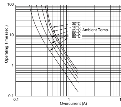
PTGL05AS6R8K3B51B0
