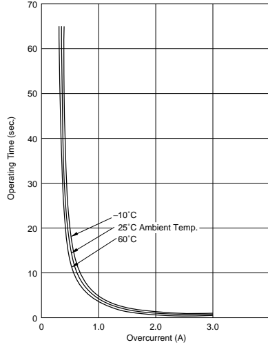
PTGL18AR6R0H8B72B0
