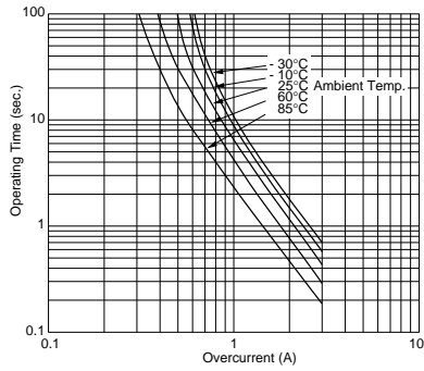
PTGL07AS3R3K3B51B0
