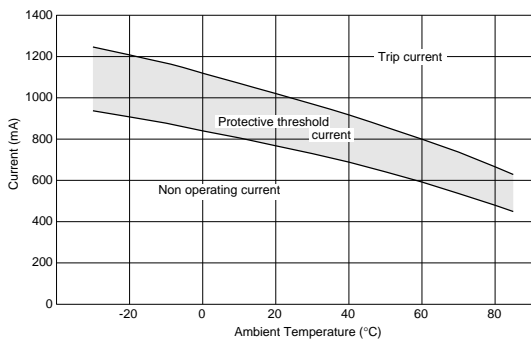
PTGL12AS1R2K3B51B0
