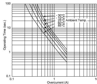
PTGL09AS120K6B51B0
