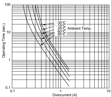
PTGL05AS100K4B51B0
