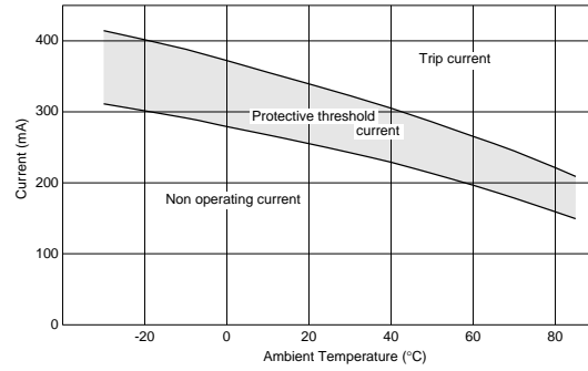
PTGL05AS6R8K3B51B0
