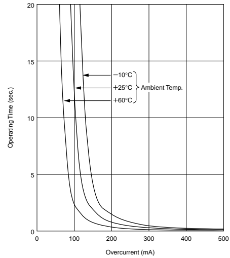
PRG21BB220MB1RK
