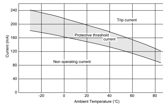
PTGL04AS220K4B51B0
