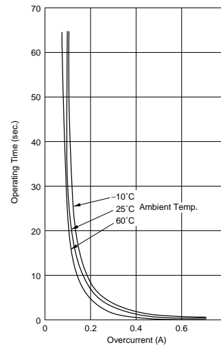
PTGL12AR150H8B72B0
