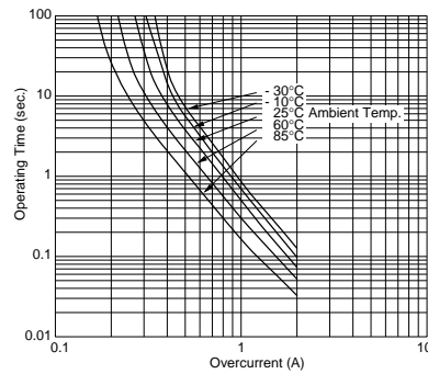
PTGL04AS100K2B51B0
