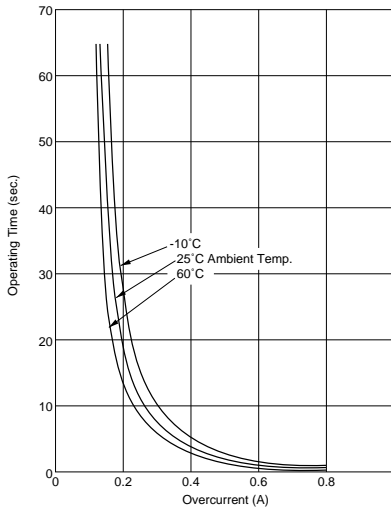
PTGL07AR700H8B52B0
