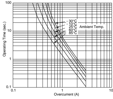
PTGL07AS5R6K4B51B0
