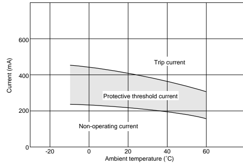
PTGL12AR150H8B72B0
