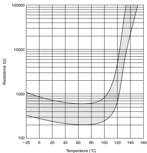
PRF_BA471Q Type
