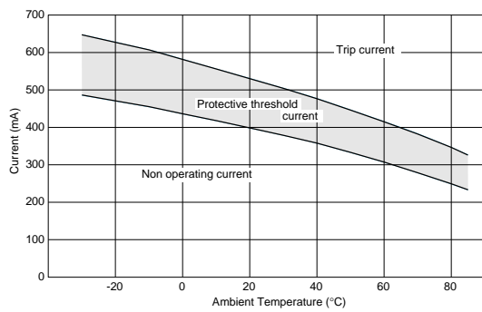
PTGL07AS3R3K3B51B0
