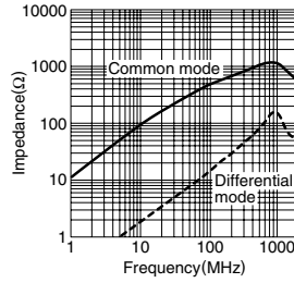
ACM3225-161-2P
