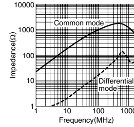
ACM3225-102-2P
