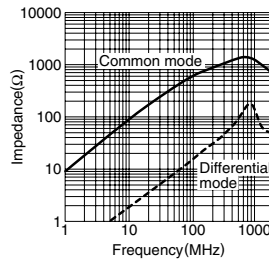
ACM3225-271-2P
