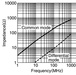
ACM2520-601-2P
