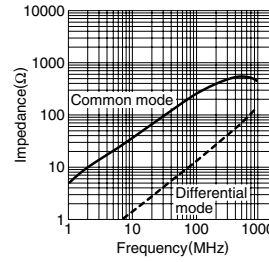
ACM3225-271-2P
