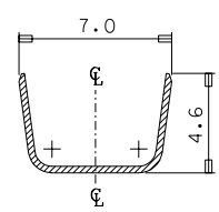
SEC' : D-D''
