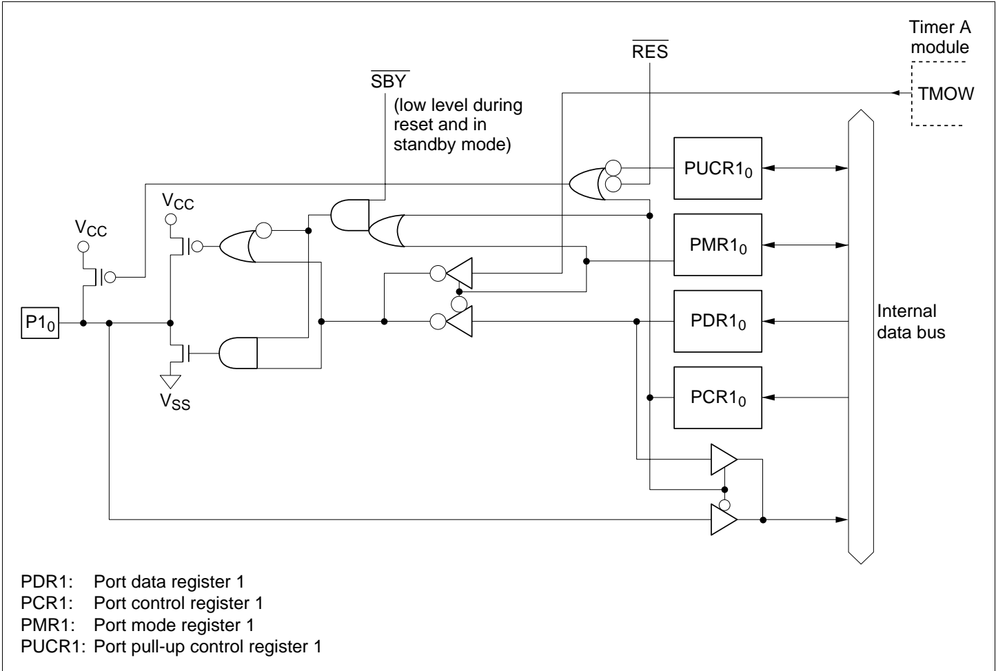
Figure C.1 (d) Port 1 Block Diagram (Pin P1 0 )
