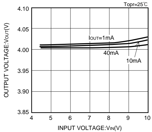
XC62HR4002 (4V)
