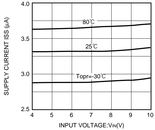
XC62HR4002 (4V)
