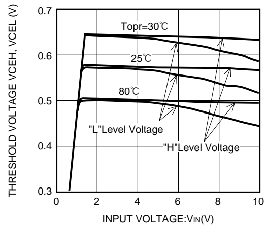
XC62HR2002 (2V)
