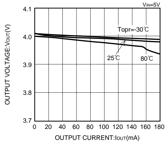
XC62HR4002 (4V)
