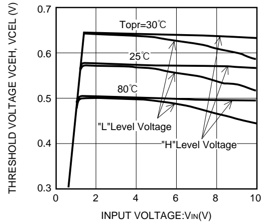
XC62HR4002 (4V)
