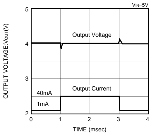
XC62HR4002 (4V)
