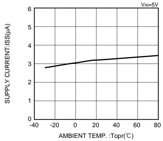
XC62HR4002 (4V)
