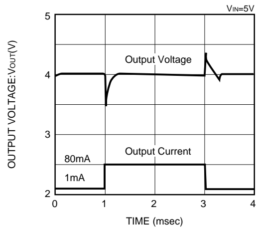
XC62HR4002 (4V)
