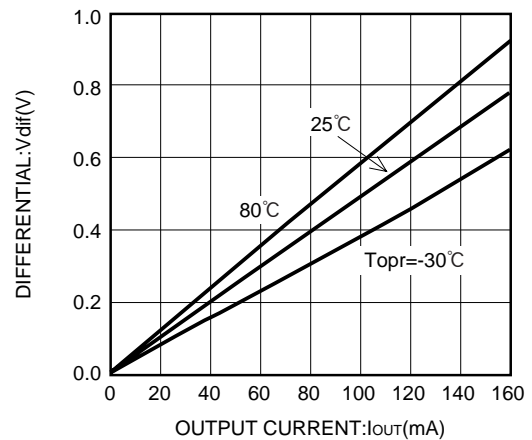
XC62HR2002 (2V)
