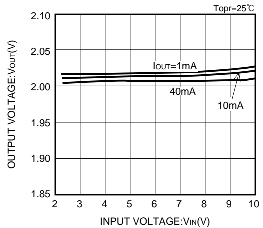
XC62HR2002 (2V)
