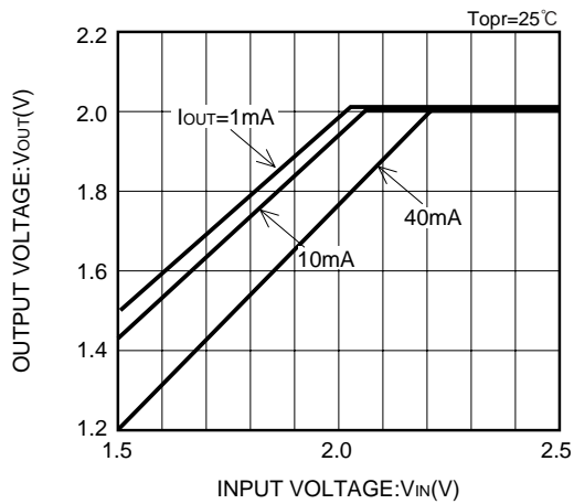
XC62HR2002 (2V)
