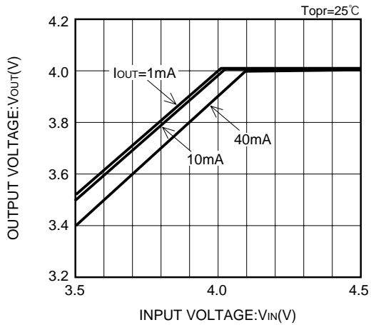
XC62HR4002 (4V)
