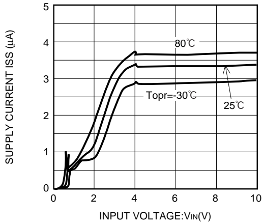
XC62HR4002 (4V)
