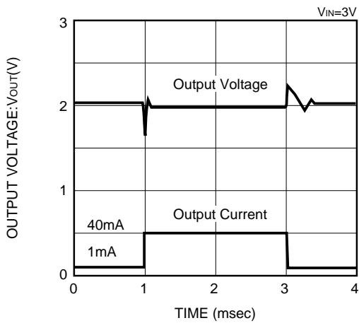
XC62HR2002 (2V)
