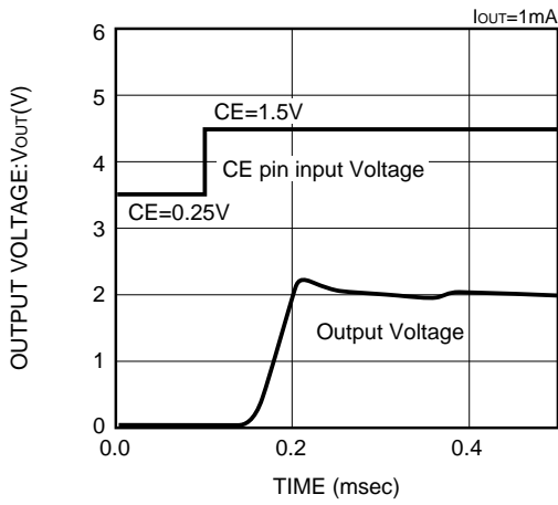
XC62HR2002 (2V)
