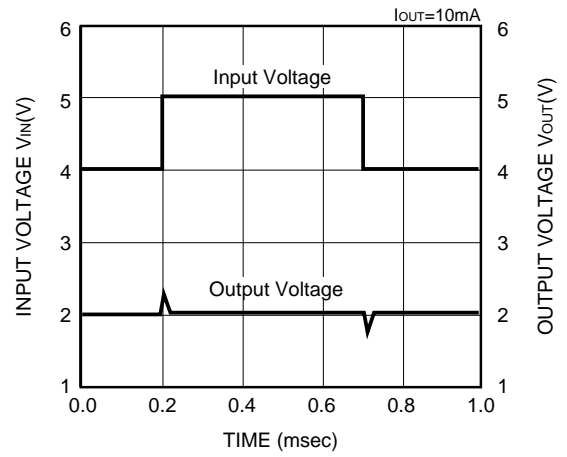
XC62HR2002 (2V)
