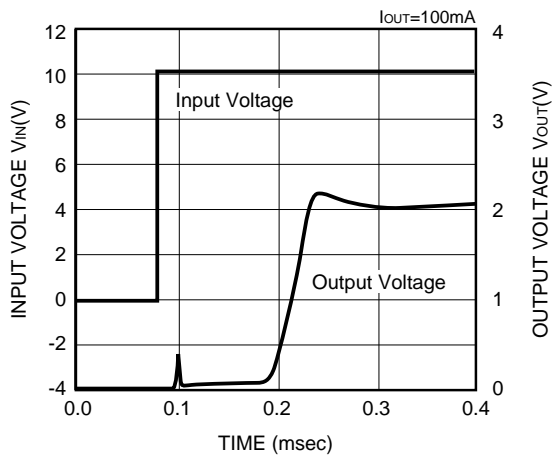
XC62HR2002 (2V)
