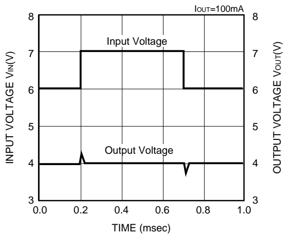
XC62HR4002 (4V)
