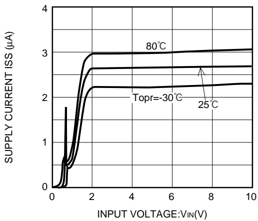
XC62HR2002 (2V)
