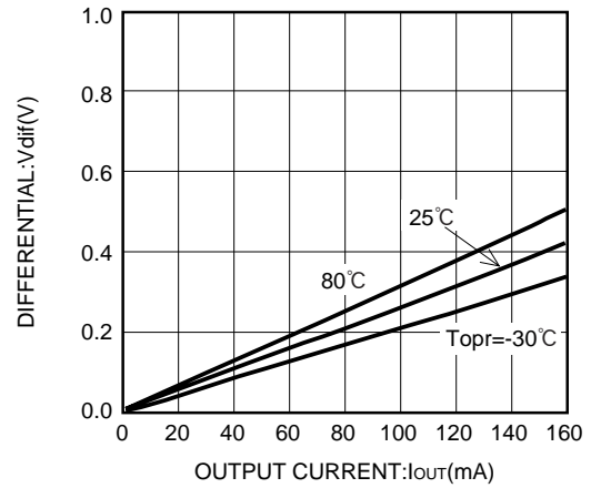
XC62HR4002 (4V)
