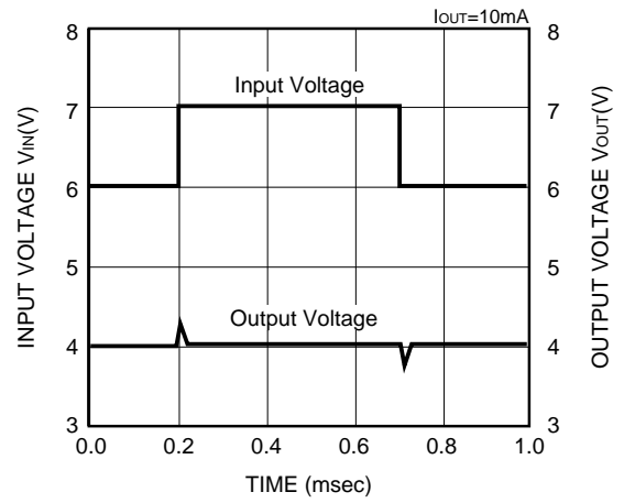
XC62HR4002 (4V)
