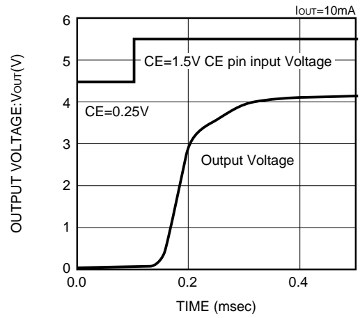
XC62HR4002 (4V)
