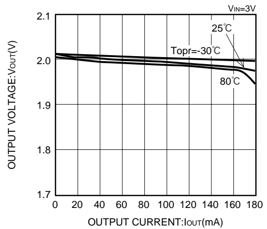
XC62HR2002 (2V)
