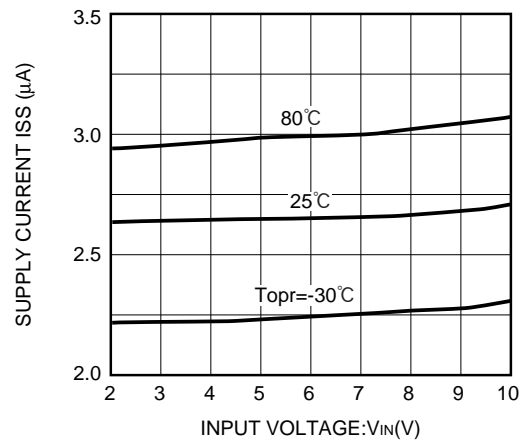
XC62HR2002 (2V)
