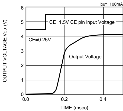
XC62HR4002 (4V)
