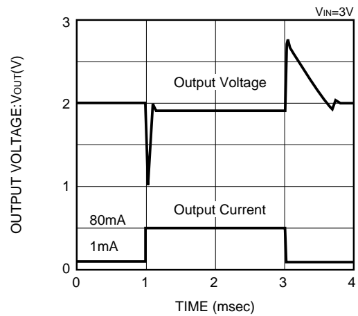
XC62HR2002 (2V)
