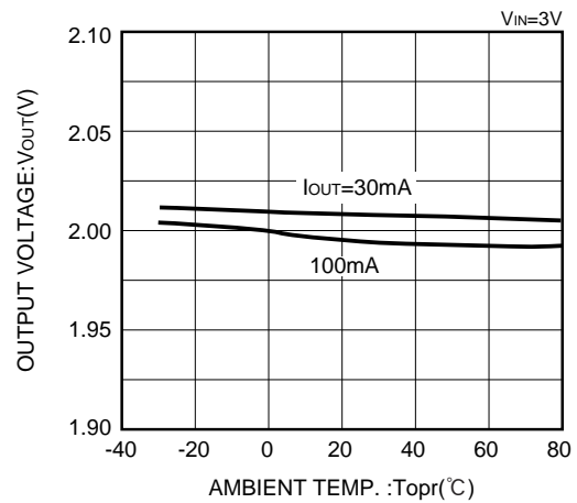
XC62HR2002 (2V)
