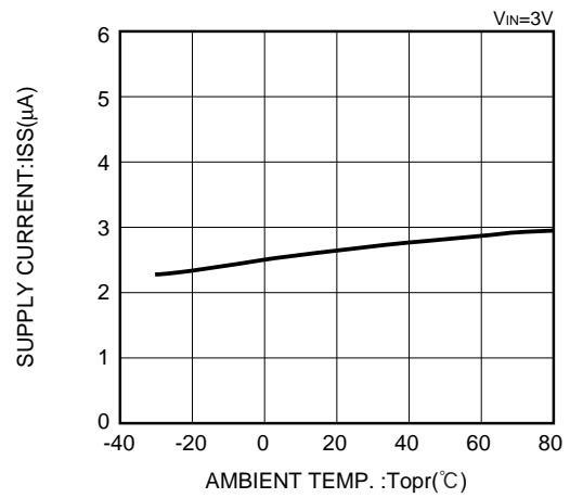
XC62HR2002 (2V)
