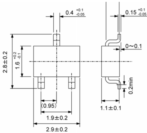
SOT-23
