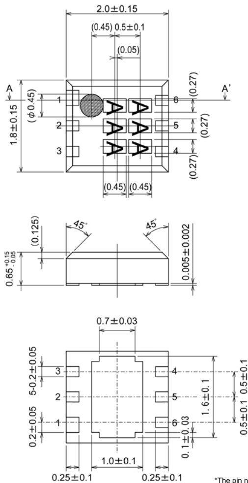
USP-6B
