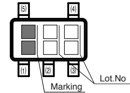
BD45XXXG/BD46XXXG : SSOP5(SMP5C2)
