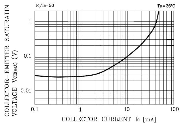
Fig. 2 V_{CE(SAT)} - I_C
