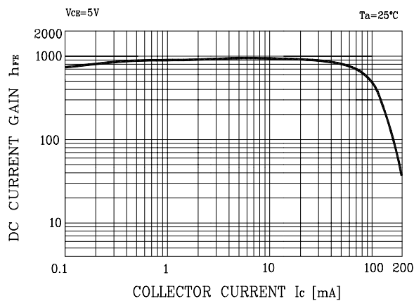
Fig. 1 h_{FE} - I_C
